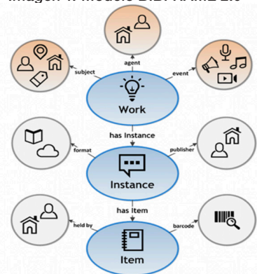
Imagen 1. Modelo BIBFRAME 2.0
