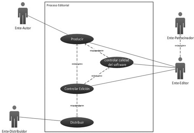
Figura 9. Modelo, nivel 7, diagrama de casos de uso para representar el proceso editorial y sus actores Fuente: Ramírez-Molina, 2022
